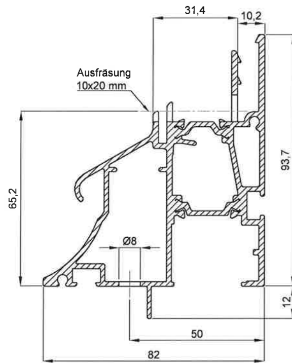
Schnitt B-B
