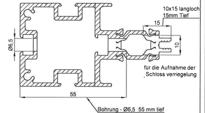
Schnitt B-B
