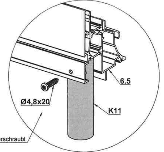
Detail Vormontage K3 (lks/re)
