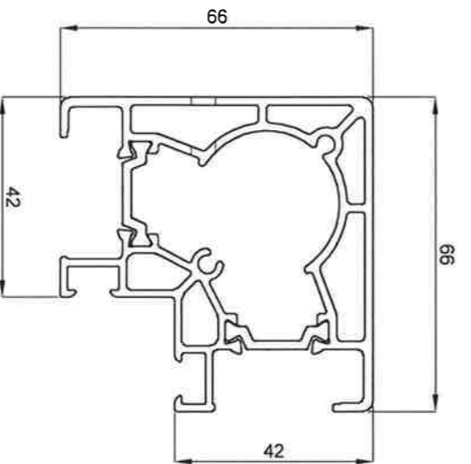
Schnitt B-B Schraubkanal auffräsen
