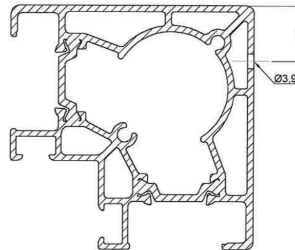
Schnitt A-A M1:1 Bohrung für Rinneneindeckelbefestigung
