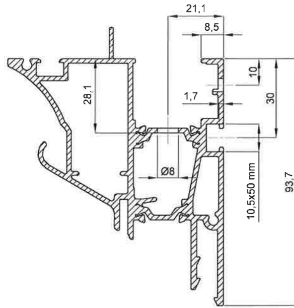
Schnitt A-A
