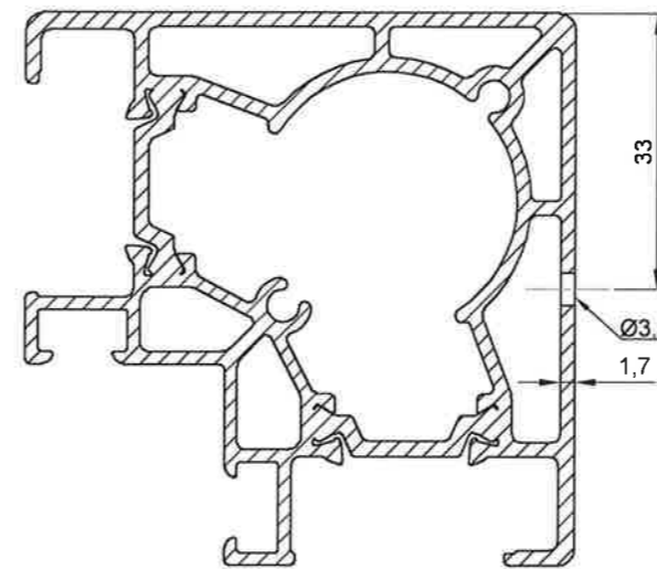
Schnitt A-A M1:1 Bohrung für Firstenddeckelbefestigung
