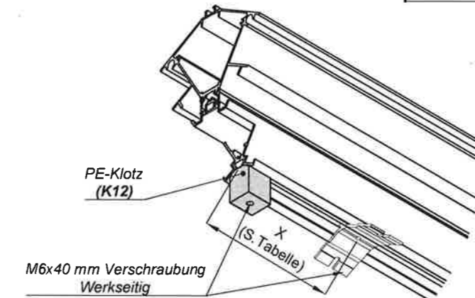
Detail A PE-Klotz anschrauben & Sprossenverbinder
