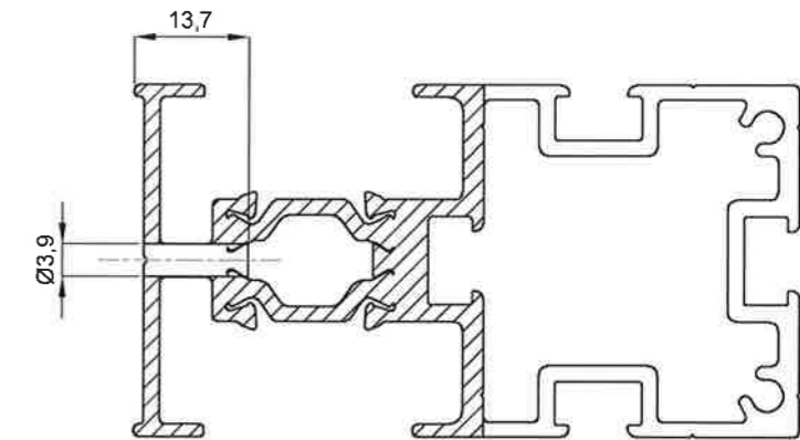
Schnitt B-B
