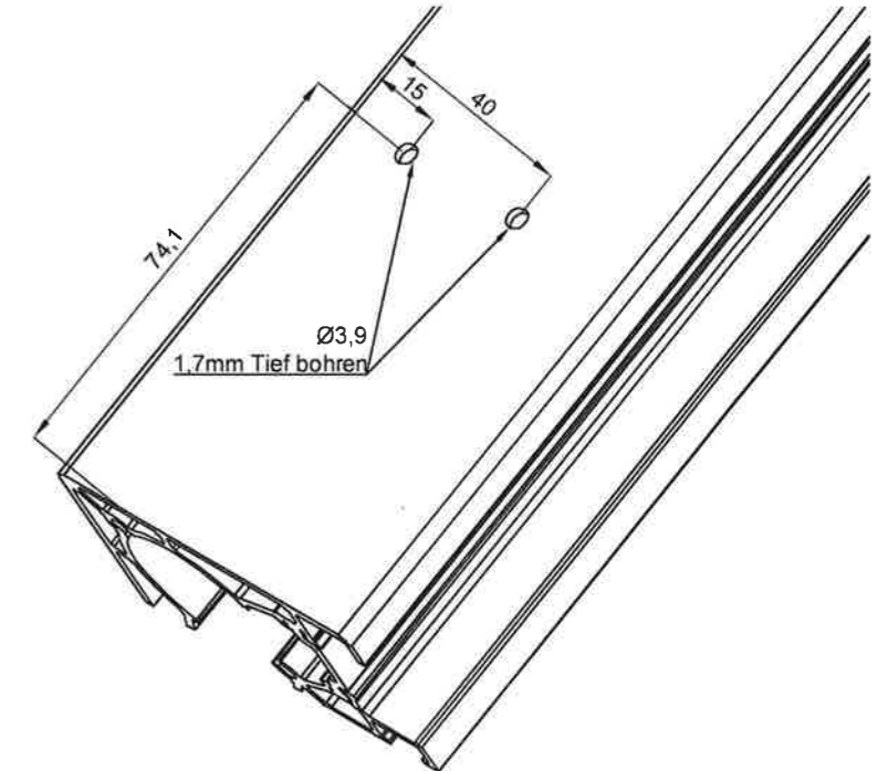
Bohrung für Rinnenenddeckel
