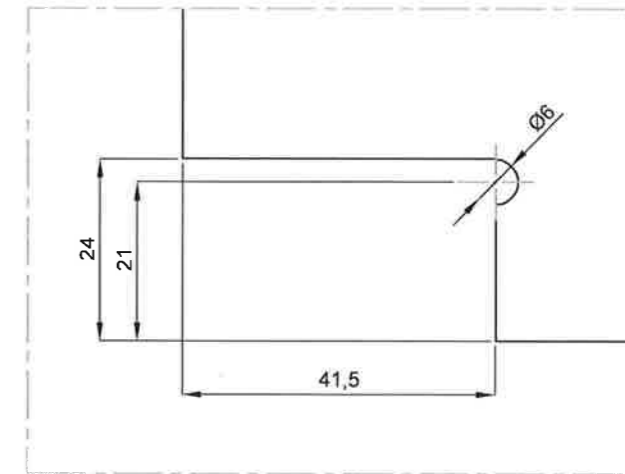
Detail A M1:1 Ausklüftung Traufenprofilseite
