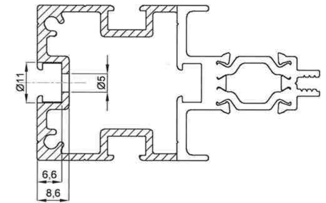
Schnitt B-B
