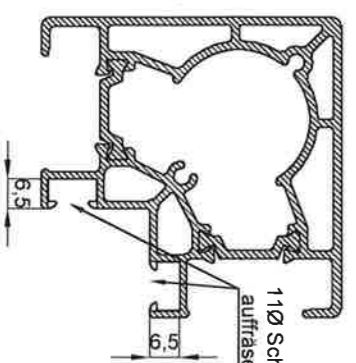
Schnitt B-B Schraubkanal auffräsen
