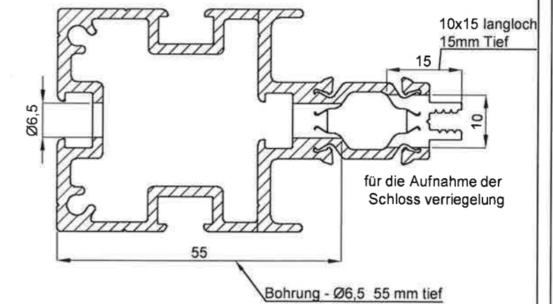
Schnitt B-B
