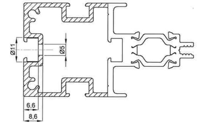
Schnitt B-B
