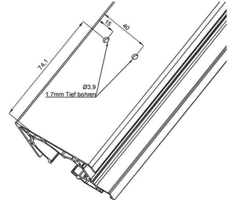
Bohrung für Rinneneindeckel
