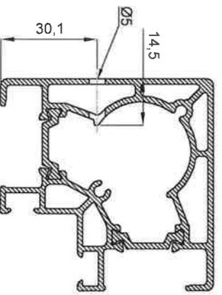
Schnitt A-A Bohrung für Fallrohrhalter
